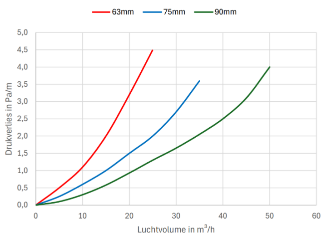
drukverlies per meter slang
